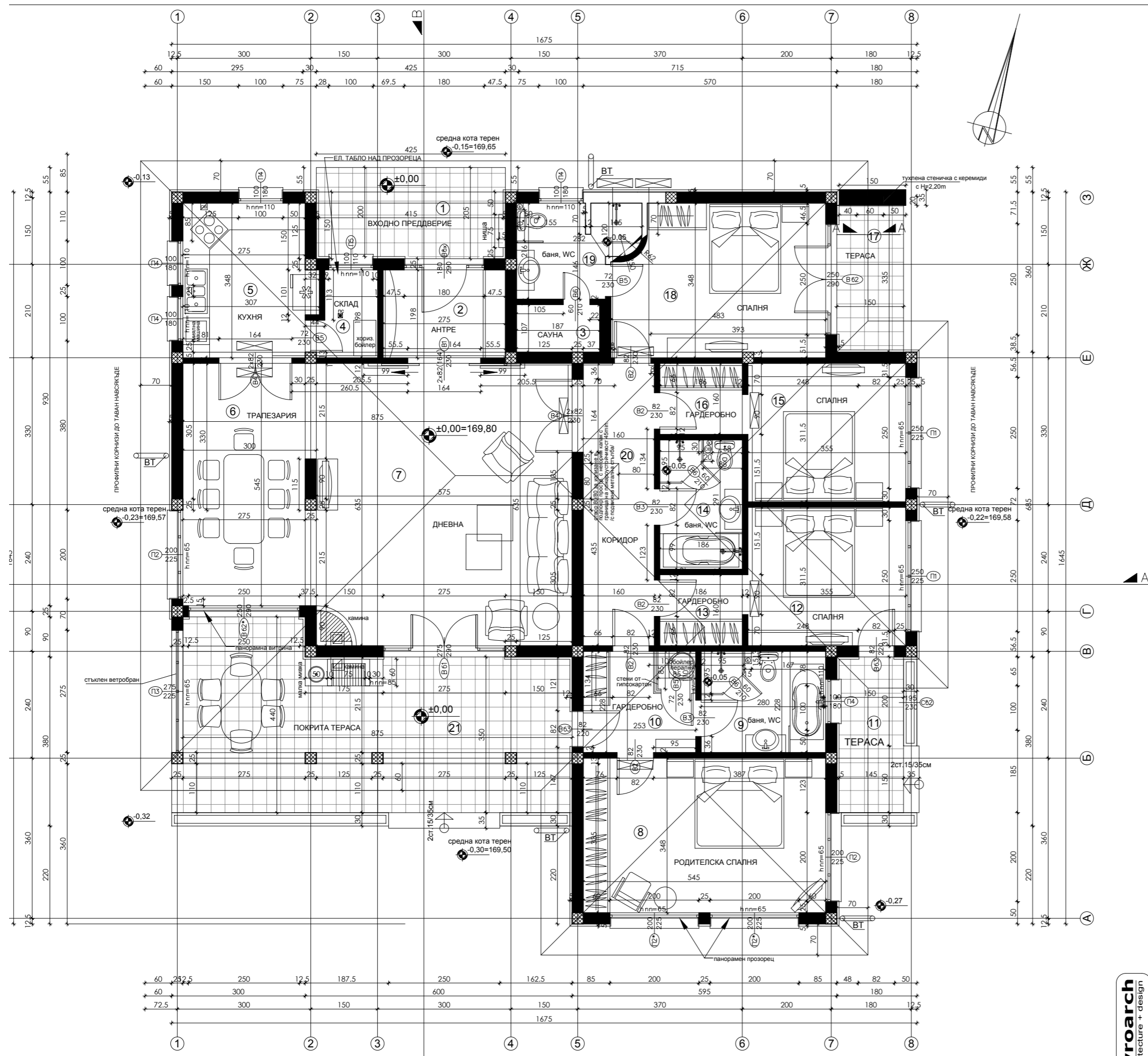
РАЗПРЕДЕЛЕНИЕ НА КОТА ±0,00
